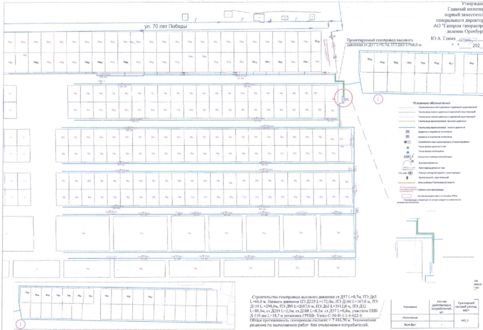
Схема сети газораспределения Газопровод к новой жилой застройке с. Палимовка
