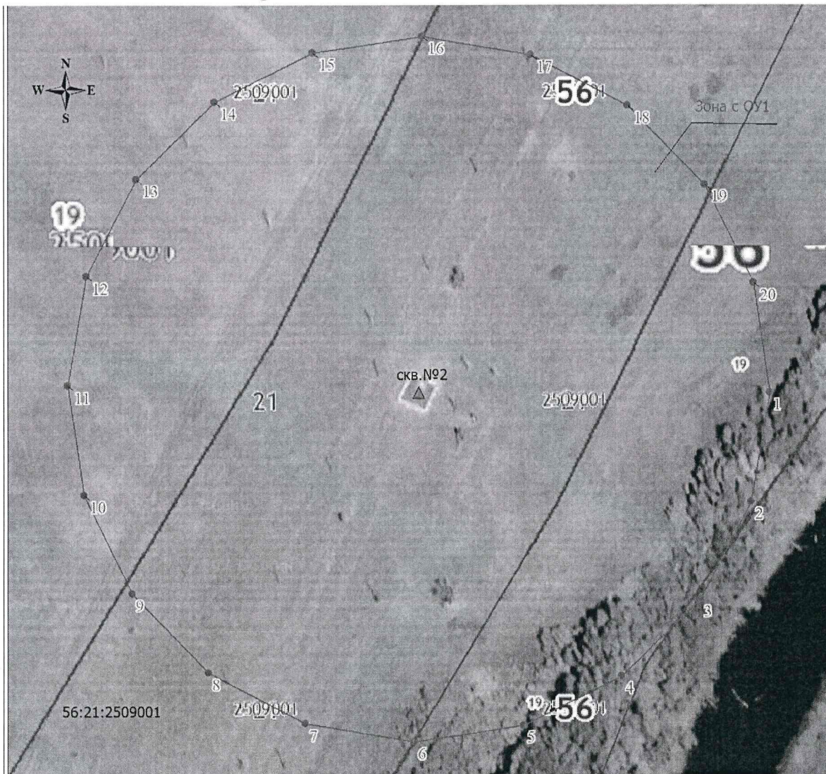
План границ II пояса ЗСО скважины № 2
